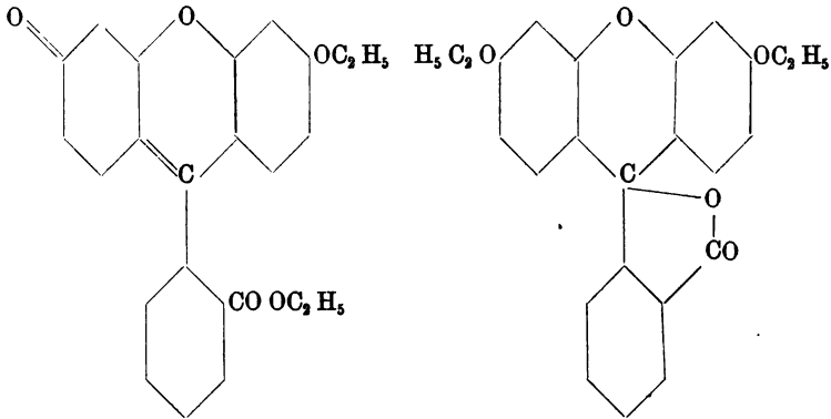
Chinoïder Diäthyläther.
